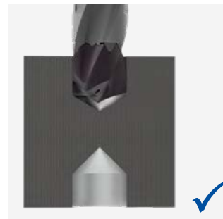
Durchbruch bei Gegenbohrung; v_f = -50\%
