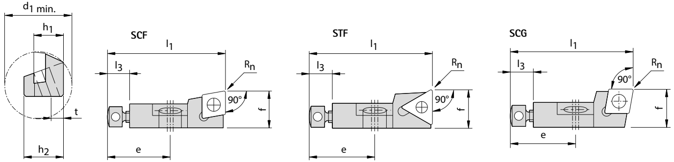
Zeichnungen in rechter Ausführung Beispiel SCFCR.
