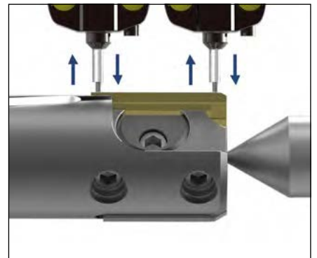
9. Ajustar las medidas de ajuste delantera y trasera en intervalos alternativos por medio de los tornillos prisioneros. Estrechamiento hacia atrás de aprox. 1 µm/mm.
