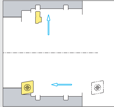
Aufbohren, Einstechen
