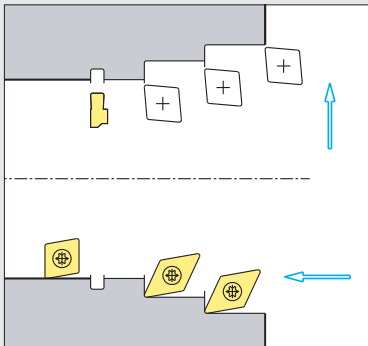
Aufbohren, Plandrehen, Einstechen (innen)
