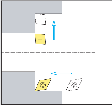
Aufbohren, Plandrehen
