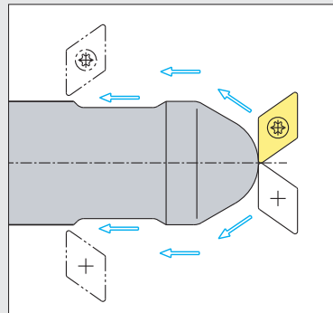
Konturdrehen, Einstechen (außen)
