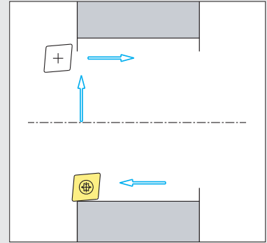
Aufbohren mit Schneidenabhebung
