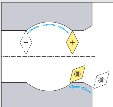
Konturdrehen (innen)
