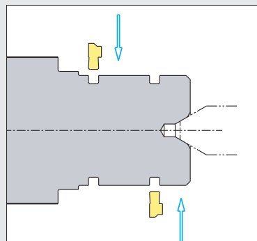
Einstechen (außen), Optional Zentrierfunktion
